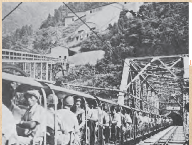
▲端出場より入坑する (昭和35年頃)
